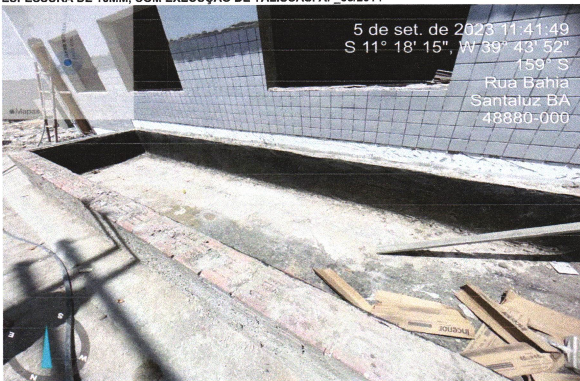
FOTO 18 - MASSA ÚNICA, PARA RECEBIMENTO DE PINTURA, EM ARGAMASSA TRAÇO 1:2:8, PREPARO MECÂNICO COM BETONEIRA 400L, APLICADA MANUALMENTE EM FACES INTERNAS DE PAREDES, ESPESSURA DE 10MM, COM EXECUÇÃO DE TALISCAS. AF_06/2014
